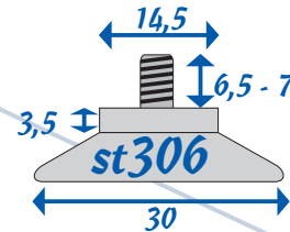
Detailzeichnung in Originalgröße
